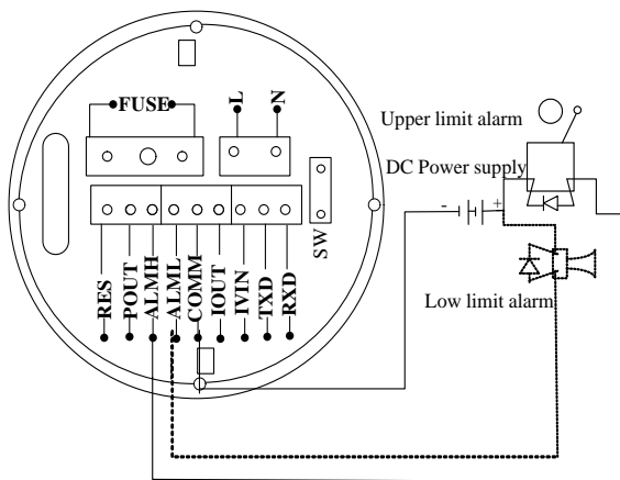
Fig 4.4.2(d) Connection of Alarm Output
